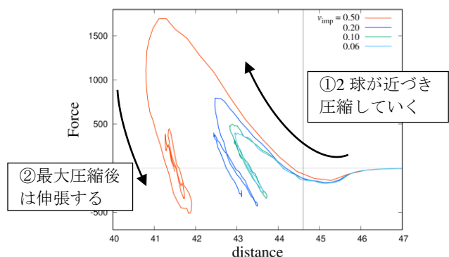
図2: 2つのモノマー重心間距離とモノマーに働く力の関係。距離は0.3405 nmで規格化されている。圧縮時と伸張時で異なる様子(ヒステリシス)が見られる。
