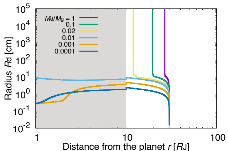
図1. 層流周惑星円盤におけるダスト(ピーク質量)の合体成長。線の色は円盤に流入するガスのダスト/ガス質量比、灰色の領域は水のスノーラインの内側を示す。Shibaïke & Mori (submitted)の図を改変。
