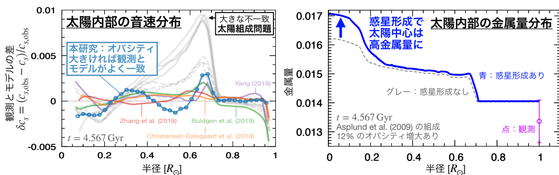
図 1: (左) 太陽内部の音速分布。実線は Asplund et al. (2009) の組成、破線は Grevesse & Sauval (1998) の組成を用いた結果。グレーは標準的な恒星進化モデル、青が本研究、それ以外の線は先行研究の結果。(右) 太陽内部の金属量分布。青・グレーの線はそれぞれ惑星形成あり・なしの結果。
