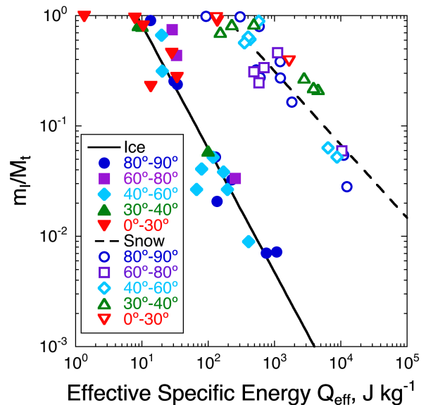
図1：規格化最大破片質量と有効エネルギー密度の関係。
