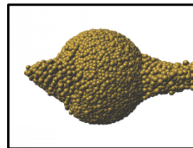
図2: 自転加速タイムスケールが1ヶ月程度で実効的摩擦角が 80^\circ の場合の、表面地滑りが起きている最中の小惑星形状。
