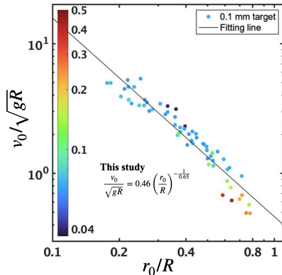
図 1：エジェクタ速度分布。色はトレーサー粒子の粒径をクレーター半径で規格化した値に対応する。
