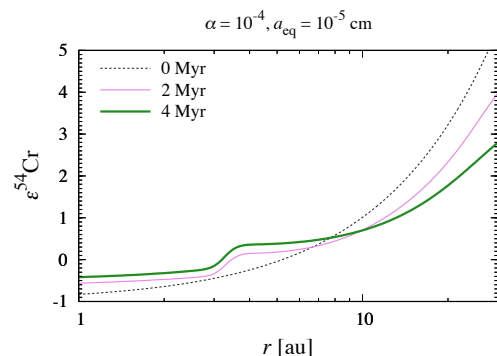
図 1 : Cr 同位体の動径方向分布[3]
