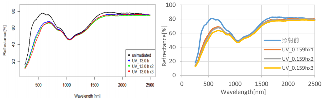
図1.左:反応が飽和したスペクトル 右:反応が飽和していないスペクトル
