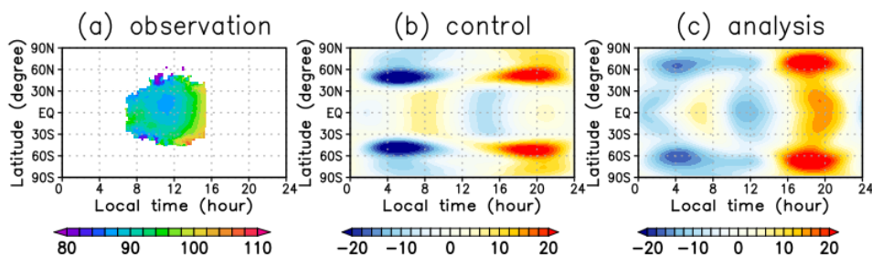
図1 2018年10-11月平均の高度70kmにおける東西風の緯度ローカルタイム図。(a) 観測、(b) 同化なし結果、(c) 同化した結果。(b, c) は帯状平均からの偏差である。
