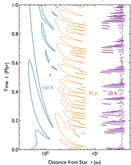
図: 熱波不安定による円盤温度分布の時間変化。3つの等温度線(160, 70, 20 K)の進化を示している。これらの線はおおむねH 2 O, CO 2 , COのスノーラインに対応する。
