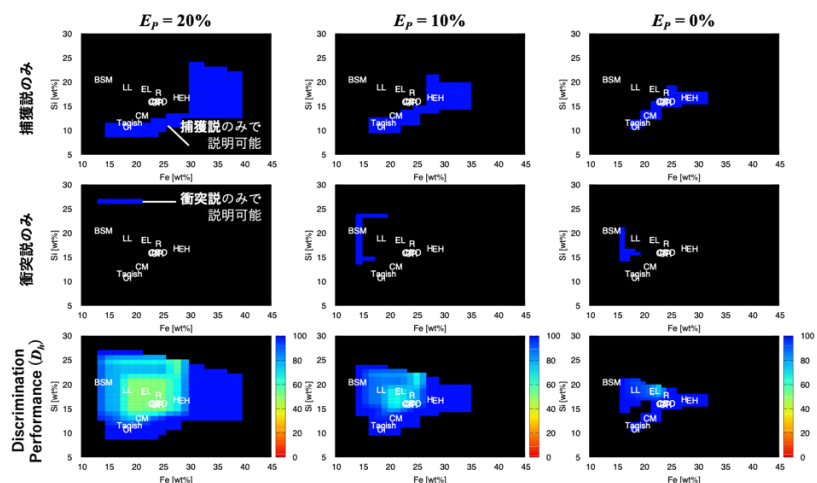
図 1 : 混合モデルに基づいて計算された Phobos のバルク組成とそれを説明できる形成仮説の関係を Fe-Si 図上で表した結果。(上段)青: 捕獲説のみにより説明可能な組成。(中段)青: 衝突説のみにより説明可能な組成。(下段)形成仮説が特定できる領域の割合(Discrimination performance)の値。
